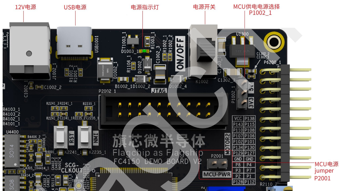
图 2. 电源接口
