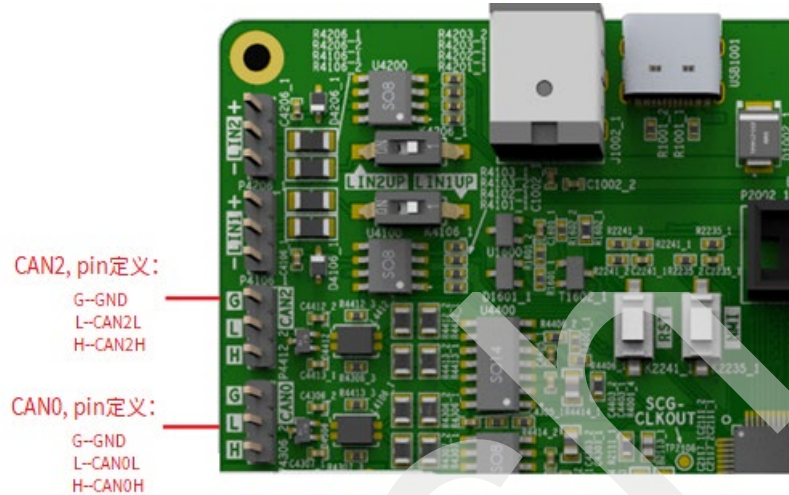
图 5. CAN 接口
