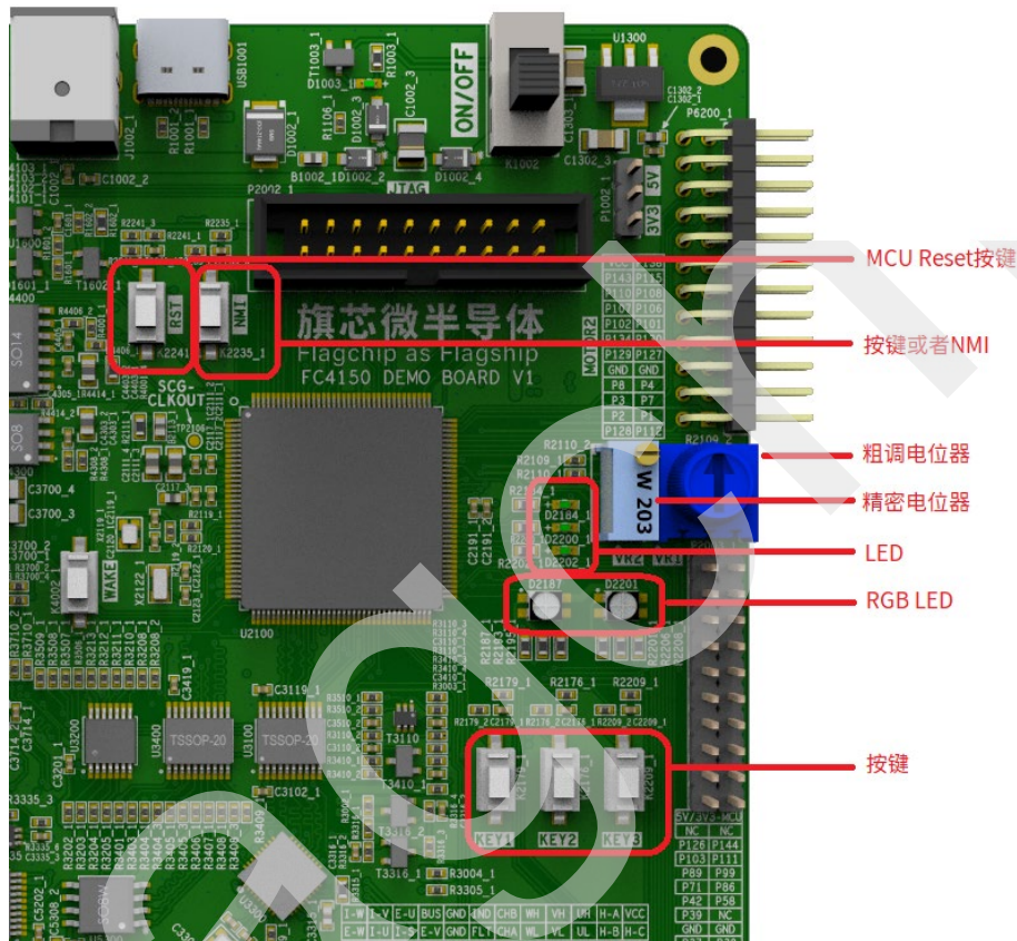
图 9. ADCs/ Keys/ LEDs 接口
